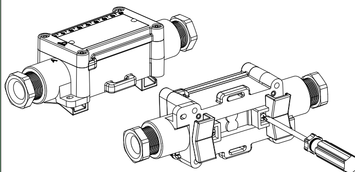
Y40伴热接线盒的组装示例
