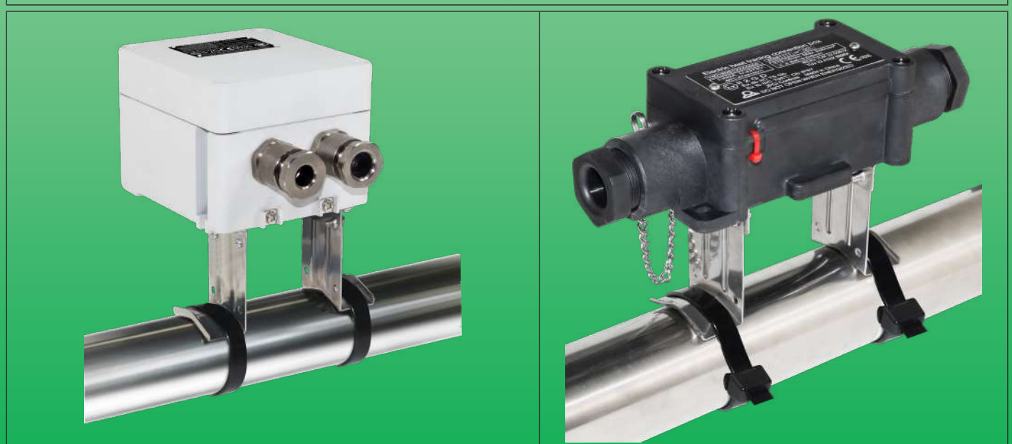
外壳140×110×90mm的组装示例 (型号 Y9)
