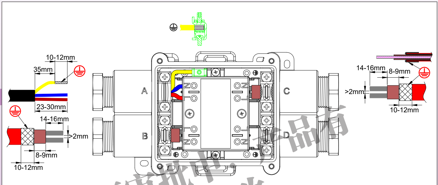
带2根发热线和一根电源电缆的型号(YB13)
