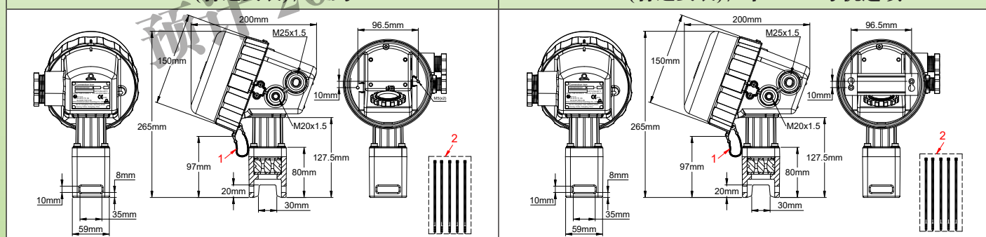
Y92 (管道安装)，空的
